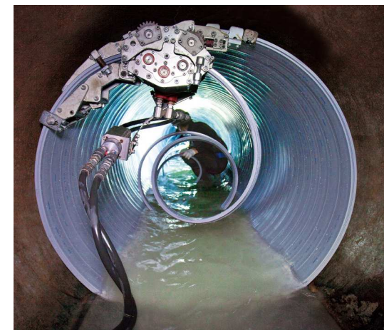
管路更生「SPR-NX工法」
